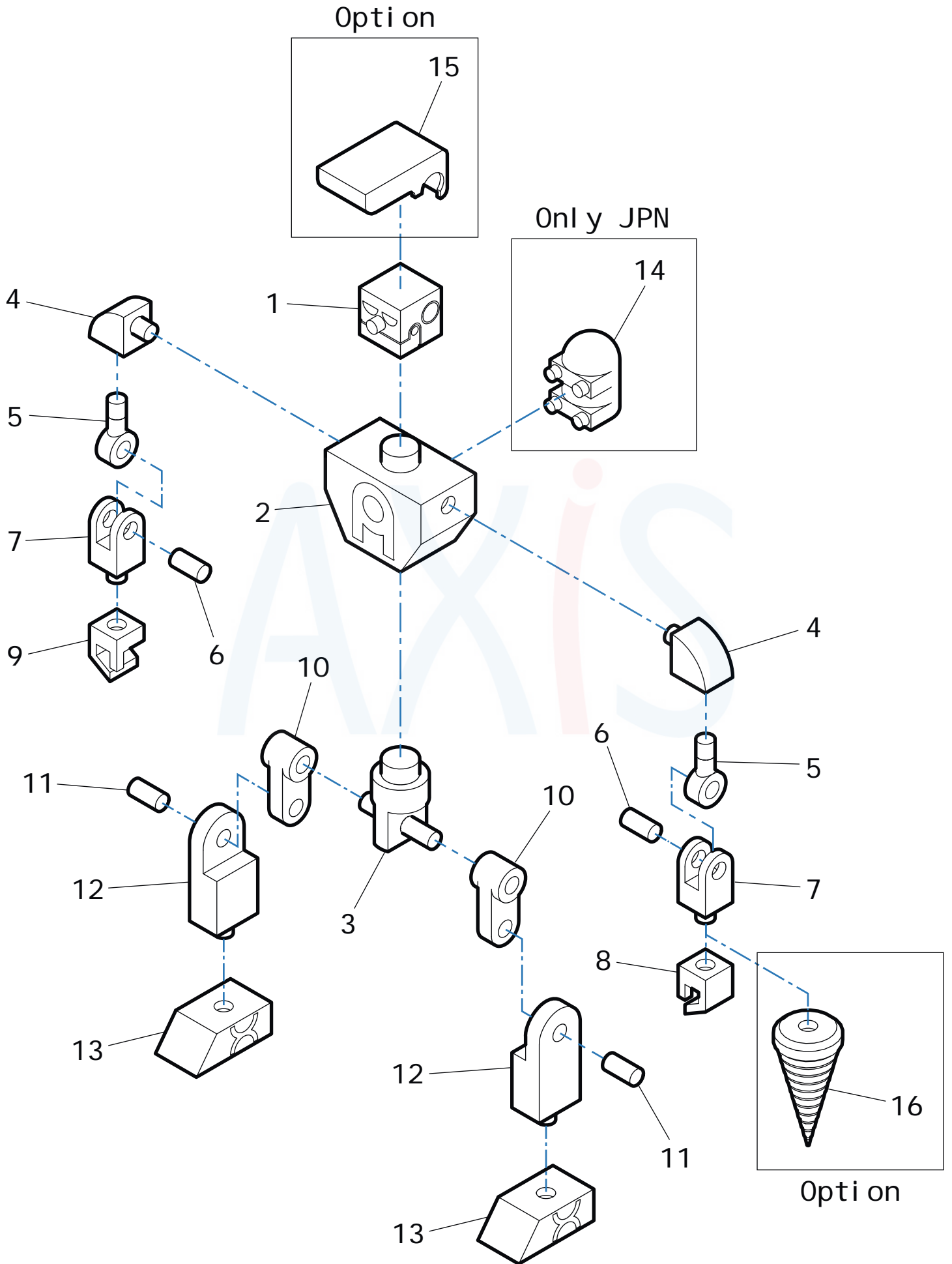
Fig. 01 AX ROBO (A type JPN)
